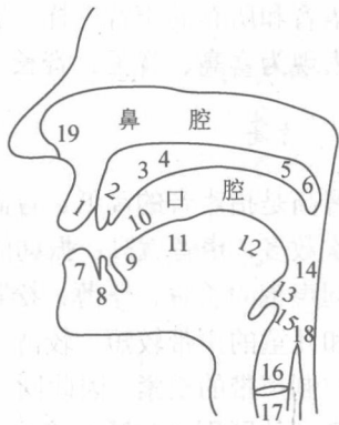
图 1-1 发音器官
