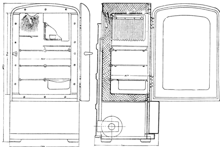
200 公升 (封閉式) 电冰箱結構图
