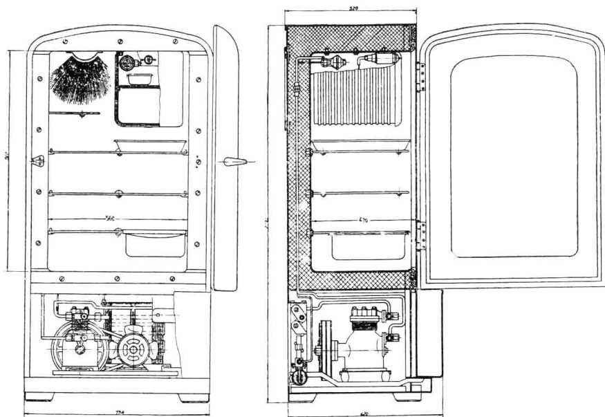
200 公升（开式）电冰箱結構图
