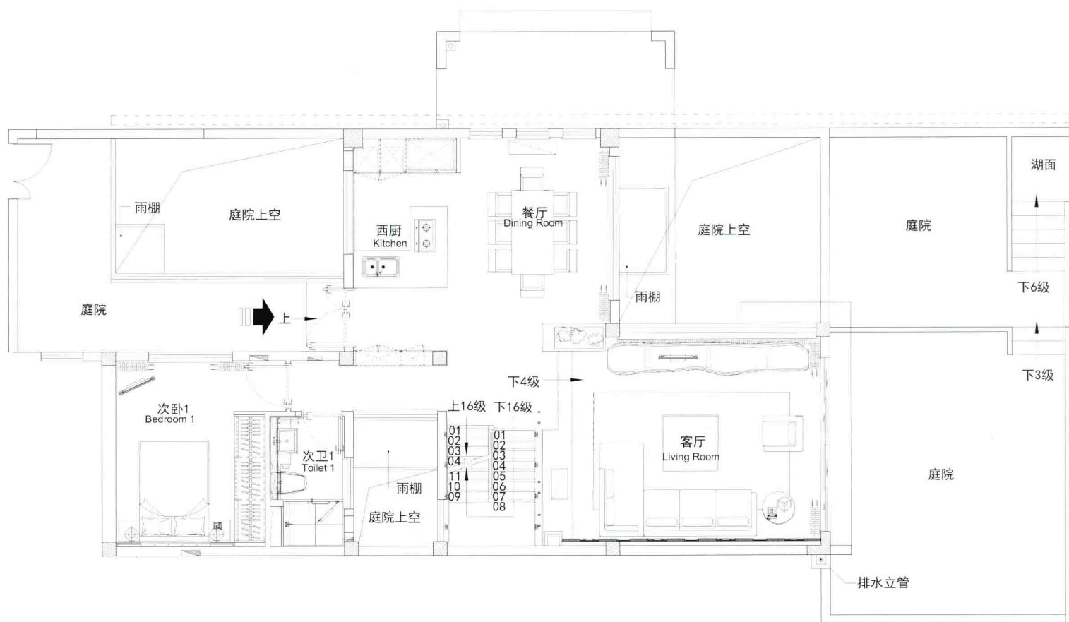
一层平面图
