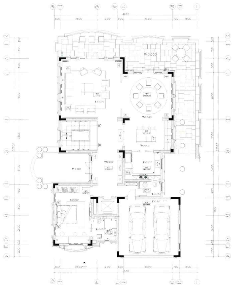
一层平面图
