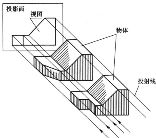
图 1—3 视图的概念
