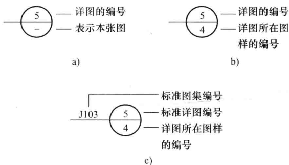
图 1—9 详图索引符号
