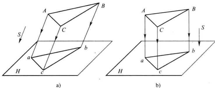
图 1—2 平行投影法
