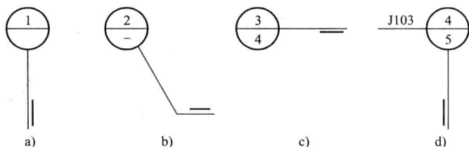
图 1—10 索引符号用于索引剖面详图
