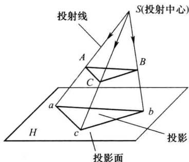
图 1—1 中心投影法
