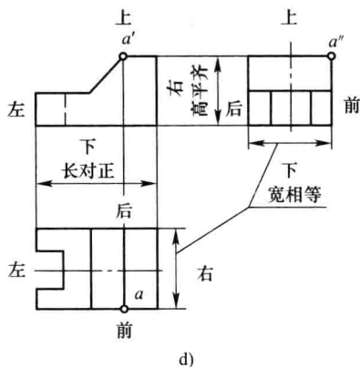
图 1—5 三视图的形成和投影规律
