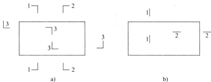
图 1—7 剖切符号
