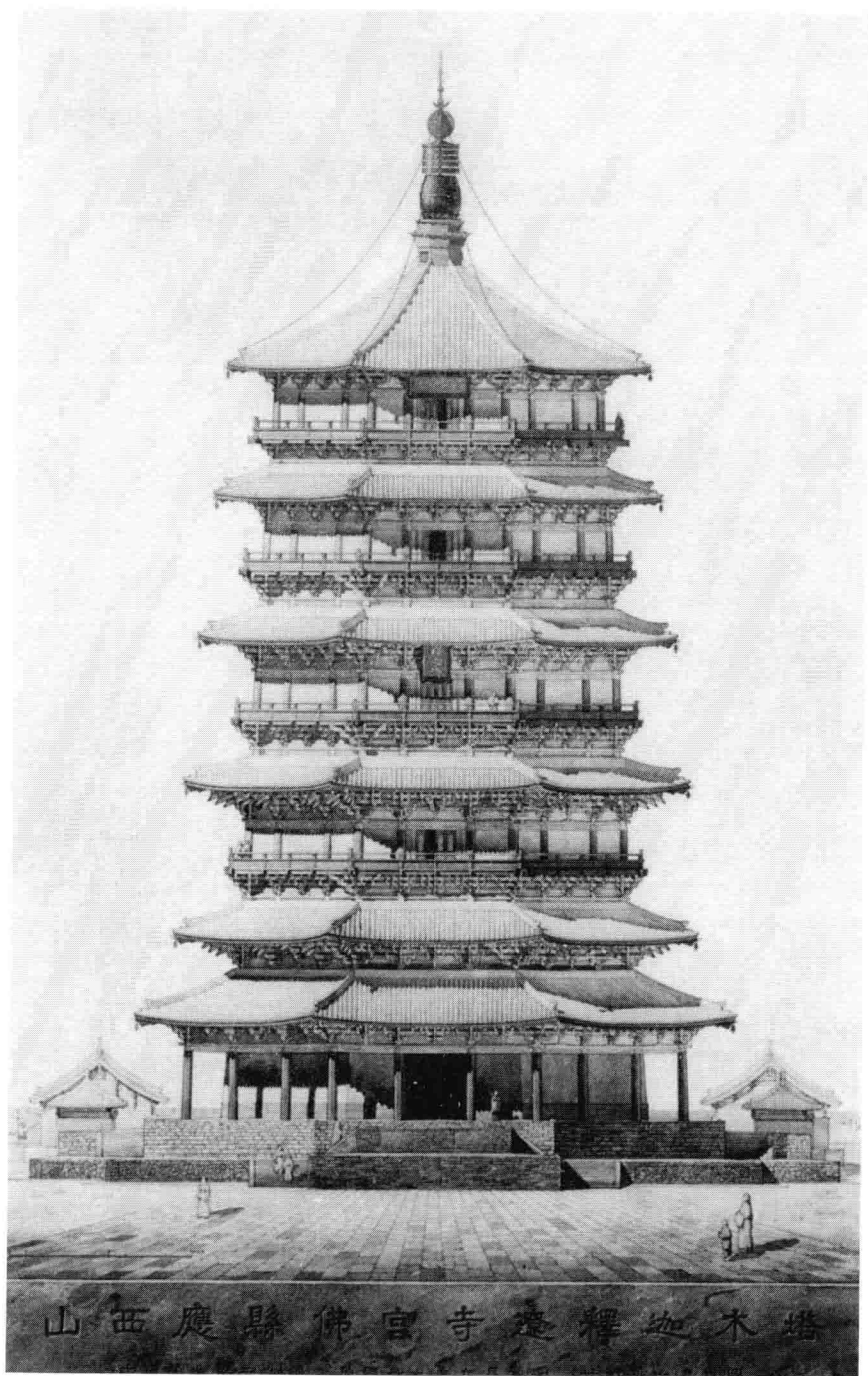
山西应县木塔梁思成手绘渲染图
