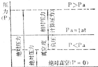
图 1-2 绝对压力和相对压力
