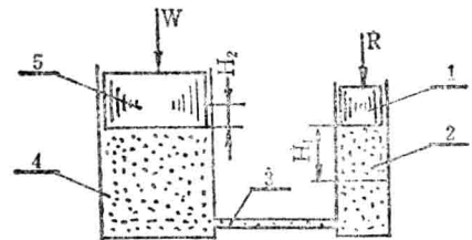
图 1-3 帕斯卡定律
