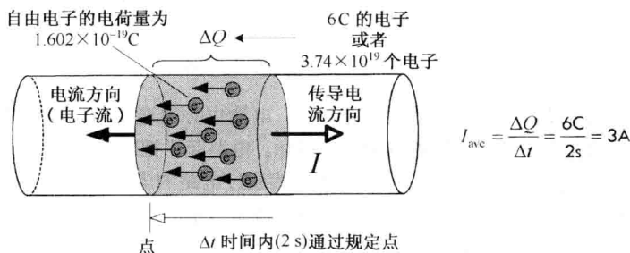
图 2.3 例 1 所示电路
