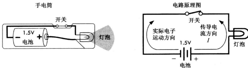
图 2.4 手电筒电路及原理图
