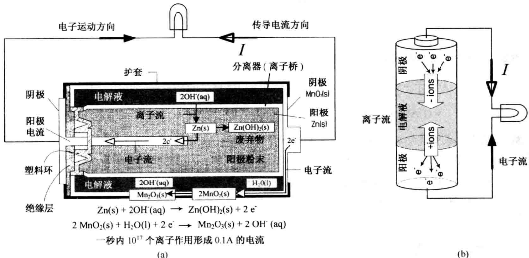
图 2.5 碱性干电池的工作原理
