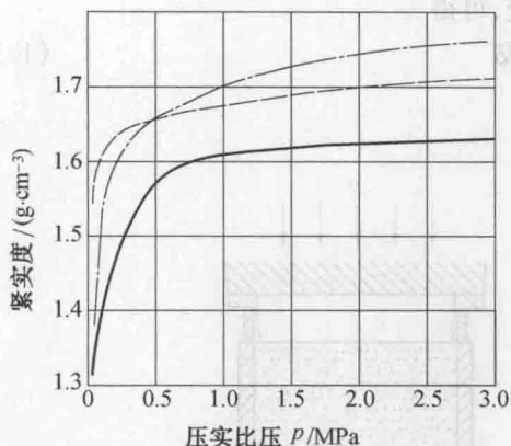
图 1.4 不同型砂的压实紧实曲线
