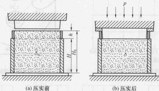
图 1.3 压实实砂
