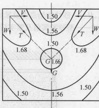
图 1.5 低速压实时砂型内的模型高紧实度区
