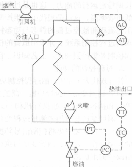
图 1-2 加热炉过程控制系统流程图
