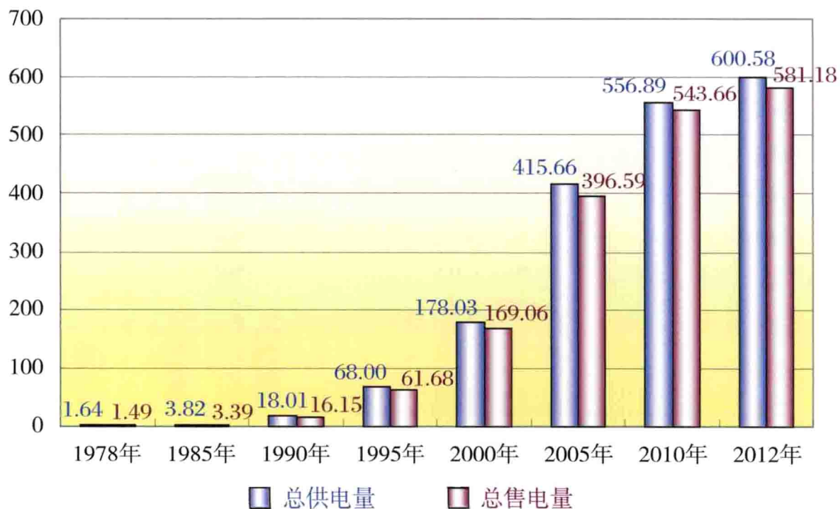
总供电量和总售电量(亿千瓦时)
