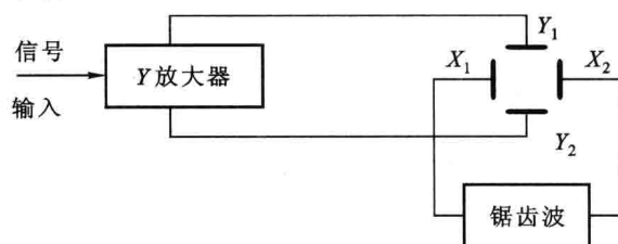
图 1.1.7 示波器工作原理图
