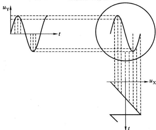
图 1.1.8 时间-波形显示原理
