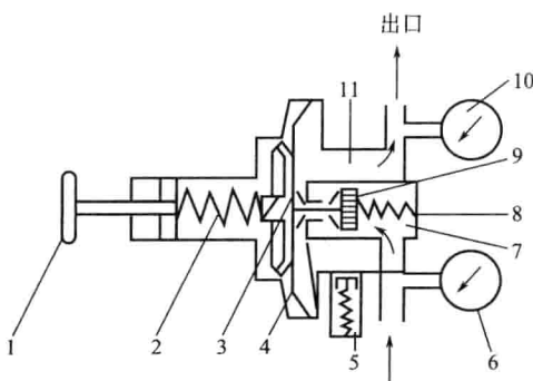
图 1-3 减压阀结构
