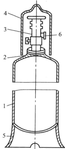
图 1-2 钢瓶剖视图
