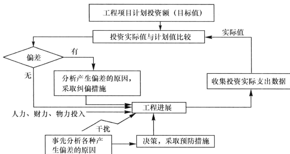
图 1-2 投资控制原理图
