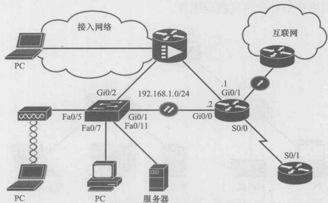
图 1-4 典型的网络示意图
