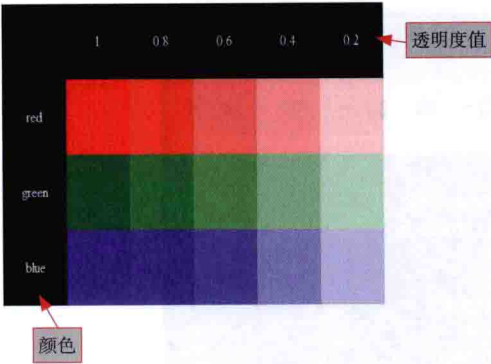
图 6-2 通过 opacity 制作渐变色块 (Chrome 25 下)
