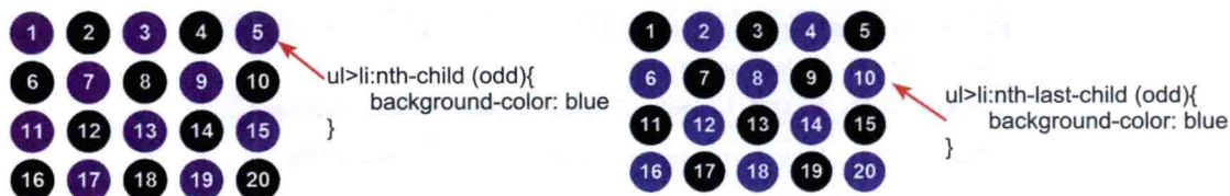
图 2-38 :nth-child(odd) 与 :nth-last-child(odd) 对比
