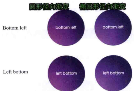
图 10-38 径向渐变圆心点在容器左下角顶点
