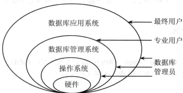
图 1.5 数据库系统层次示意图
