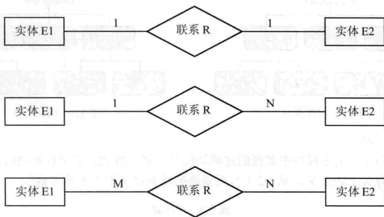
图 1.1 两个实体的三类联系
