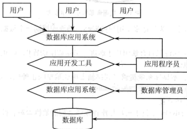
图 1.4 数据库系统 (DBS)
