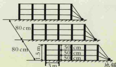
篱壁架
