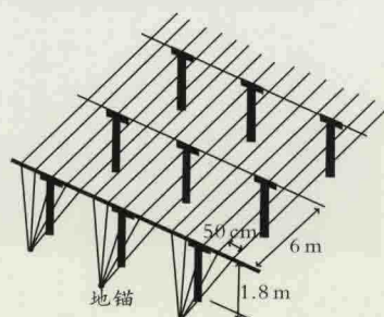
大棚硬架
