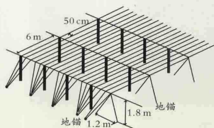
大棚软架
