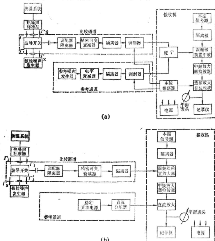
图 1 热噪声标准及校准系统方框图
