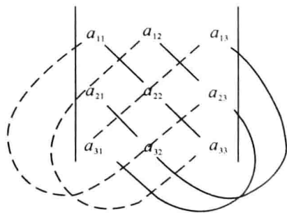
图 1.1 三阶行列式的对角线法则
