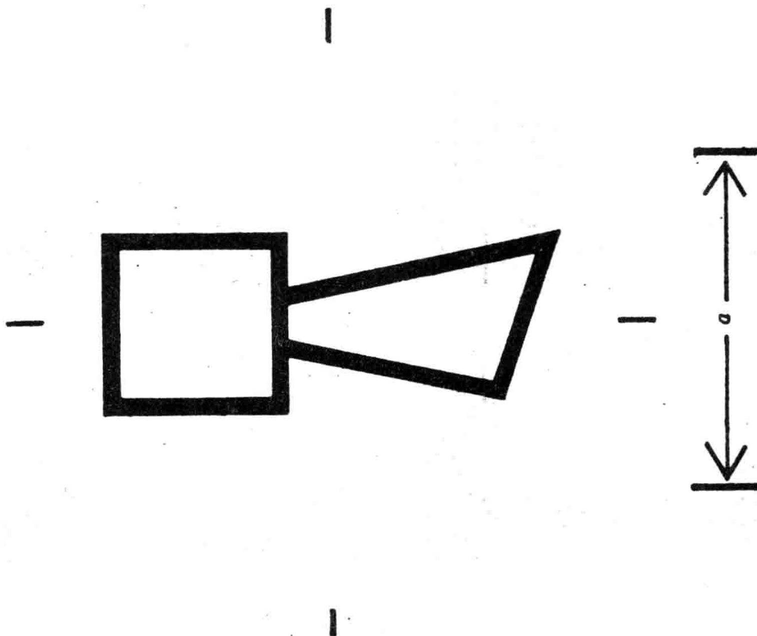
图 5 标有可见中心线符号的例子
