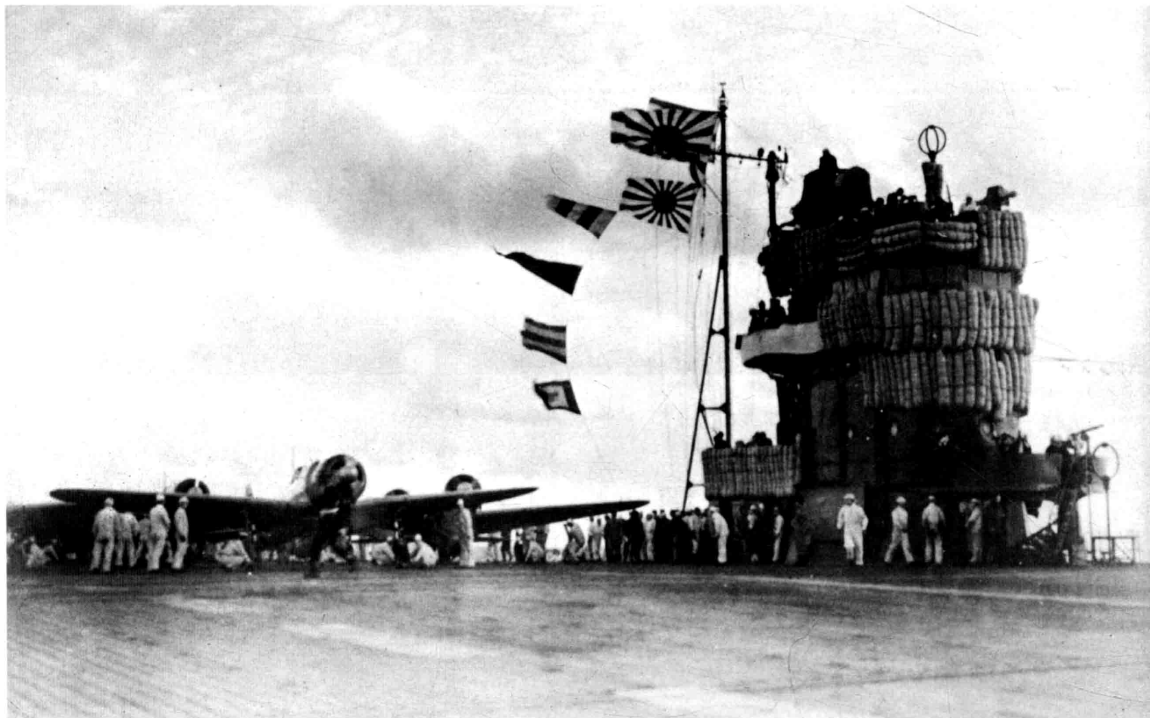
12月7日（夏威夷時間），準備起飛第二攻擊波的航空母艦「赤城」號。低矮的桅桿上戰鬥旗飄揚，左側第一架為艦戰隊長進藤三郎大尉的「零式21型」戰鬥機。
