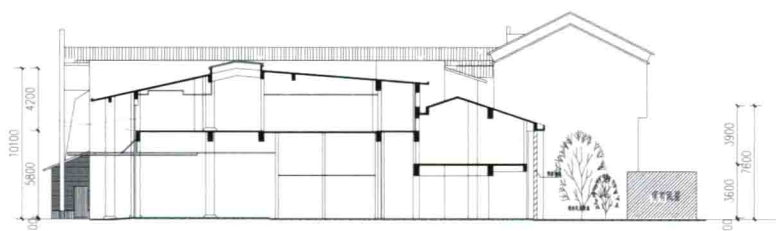
八、九号楼剖面图
