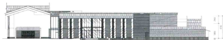
八、九号楼北立面图
