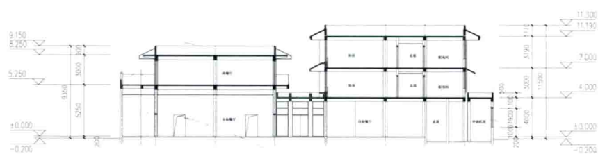
十、十二号楼剖面图1
