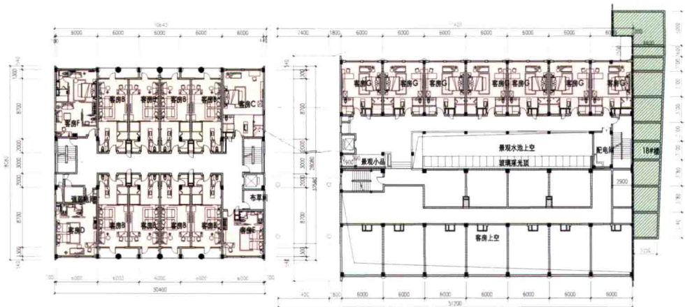
十六、十七号楼二层平面图
