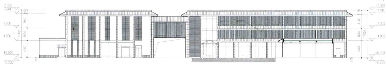
十、十二号楼南立面图
