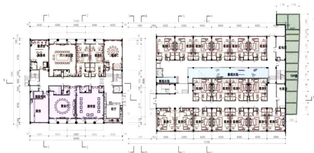
十六、十七号楼一层平面图
