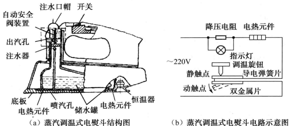
图 1.1 蒸汽调温式电熨斗
