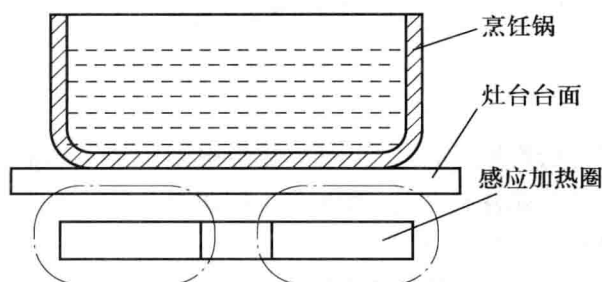
图 1.2 高频电磁灶的结构示意图
