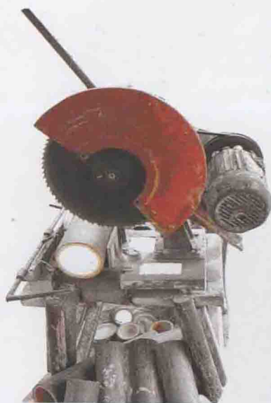
断竹机
