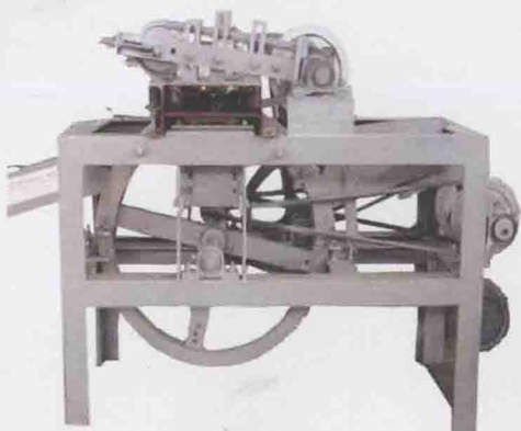
竹签成型机
