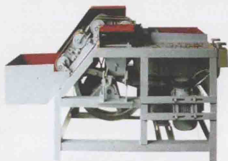
竹筷削尖成型机
