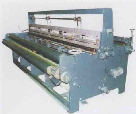
凉席编织机
