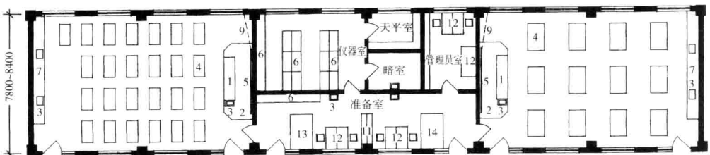
(b) 生物、物理实验室平面布置
