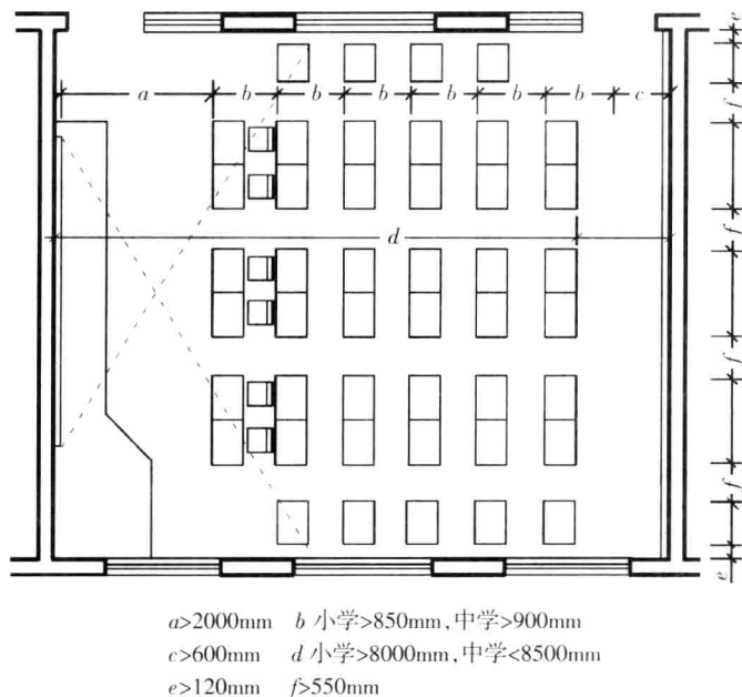
图 1.6 教室课桌椅布置及相关尺寸
