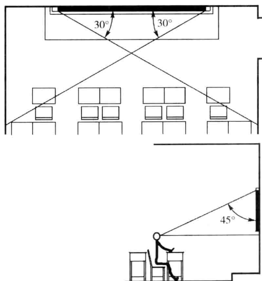
图 1.7 教室座位的视角
