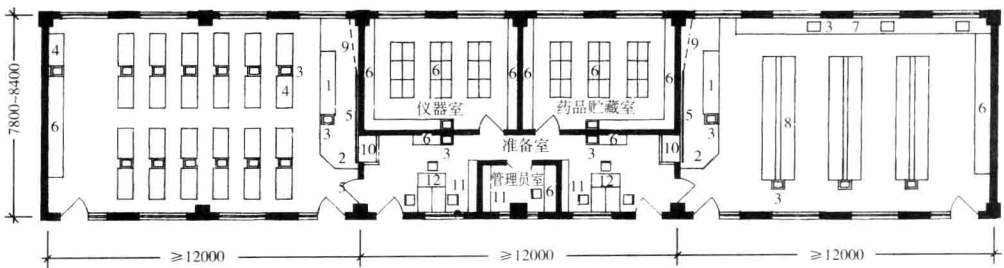
(a) 化学实验室平面布置
