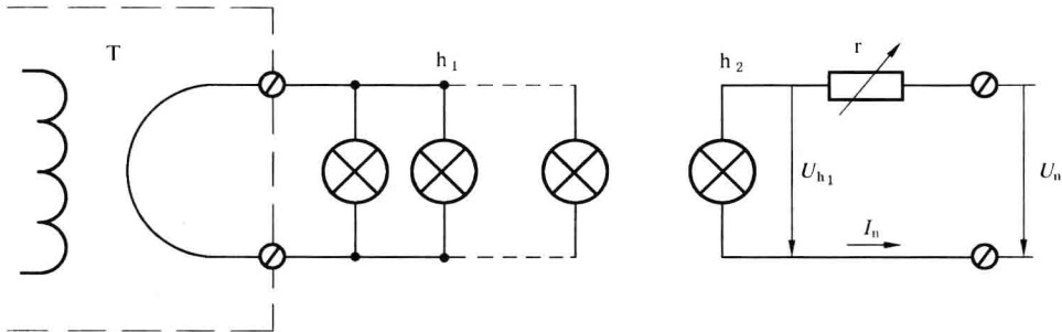
图 5 可调电感的举例
