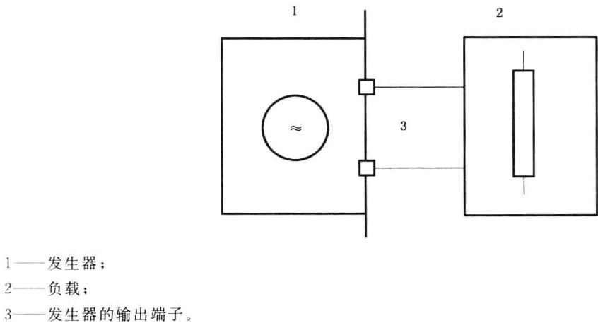
图 1 输出功率的定义
