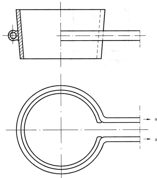
图 3 功率测量用水电阻器举例
