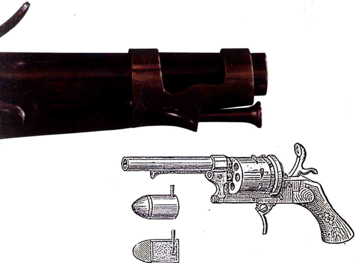
★ 早期的左轮手枪和枪弹示意图
