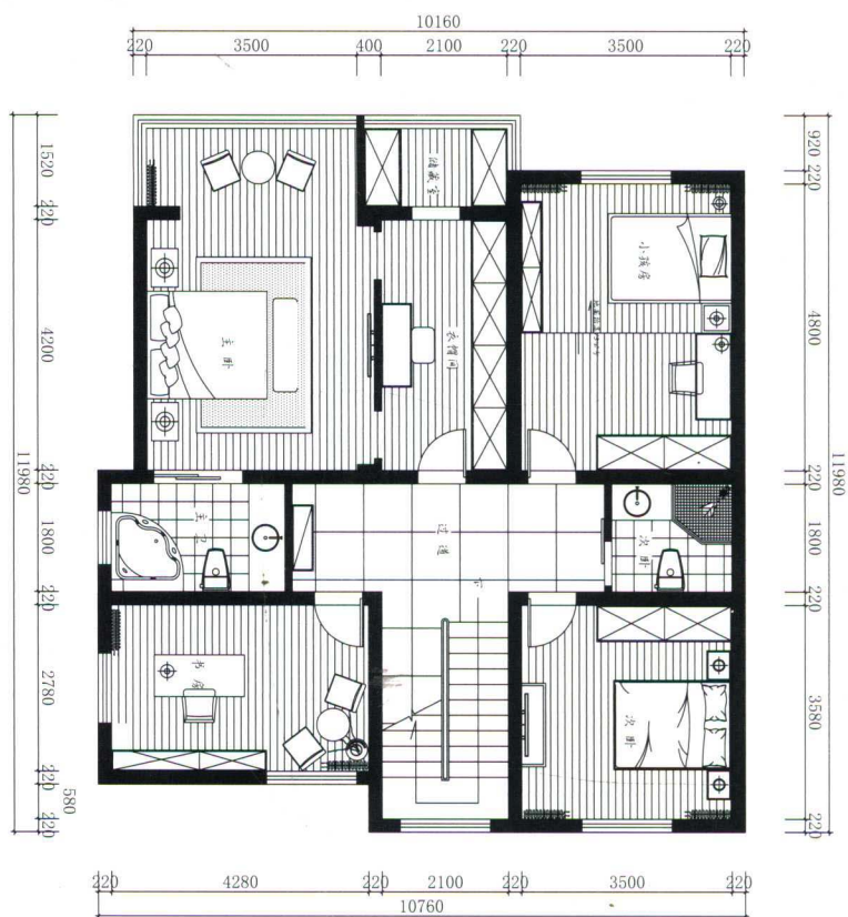
平面图 Plan
