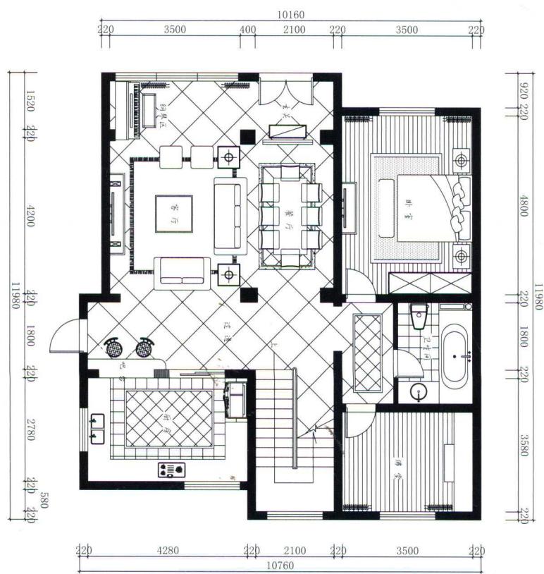
平面图 Plan
