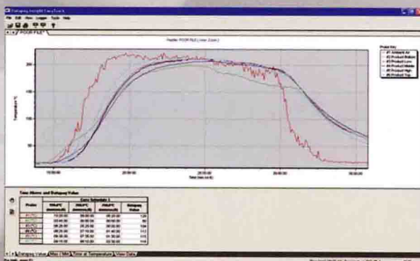
图2A: 示例故障炉温度曲线图表
