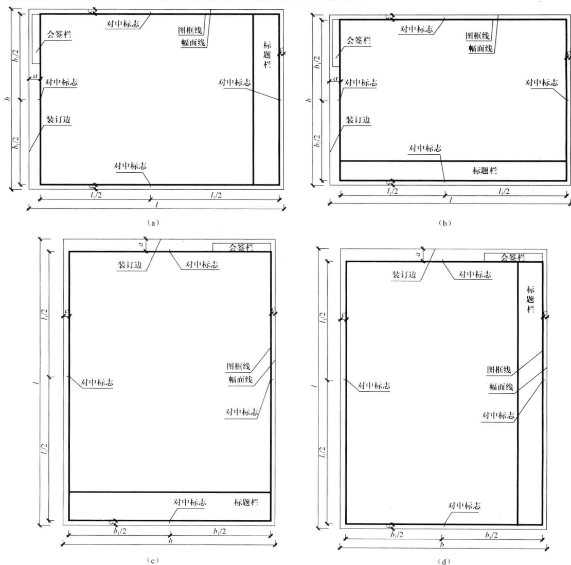
图 1-1 图纸幅面
