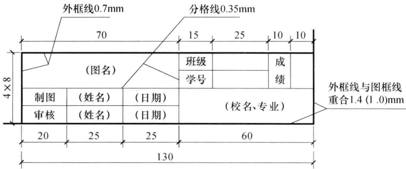
图 1-3 学习阶段的标题栏 (a) 标题栏一；(b) 标题栏二
