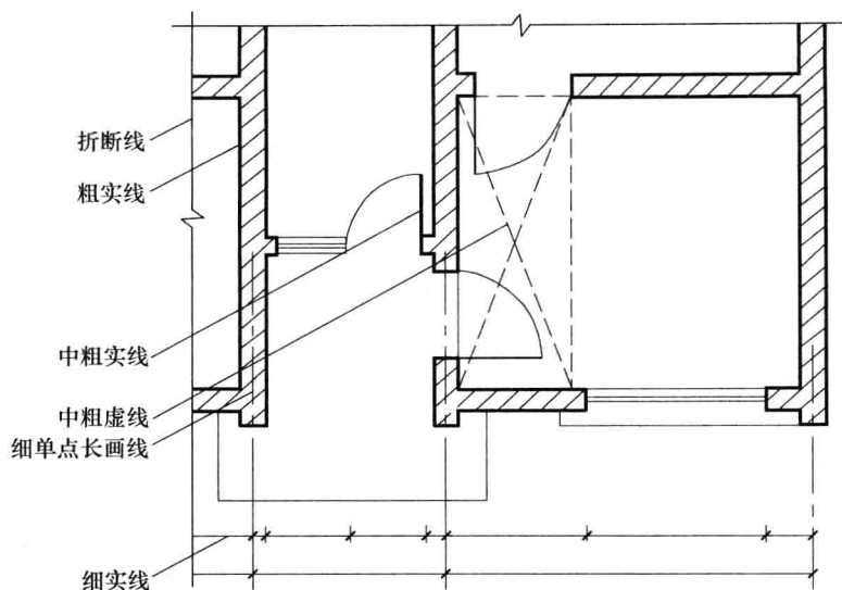
图 1-4 图线的应用
