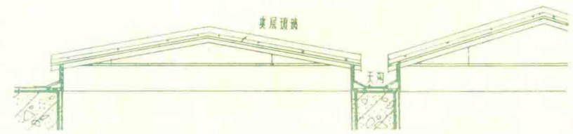
上海宾馆透光雨罩
