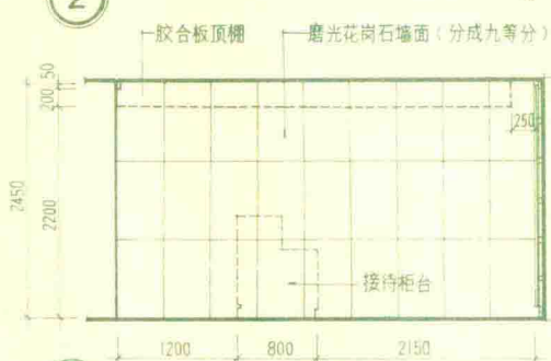
门厅接待处详图(一)
