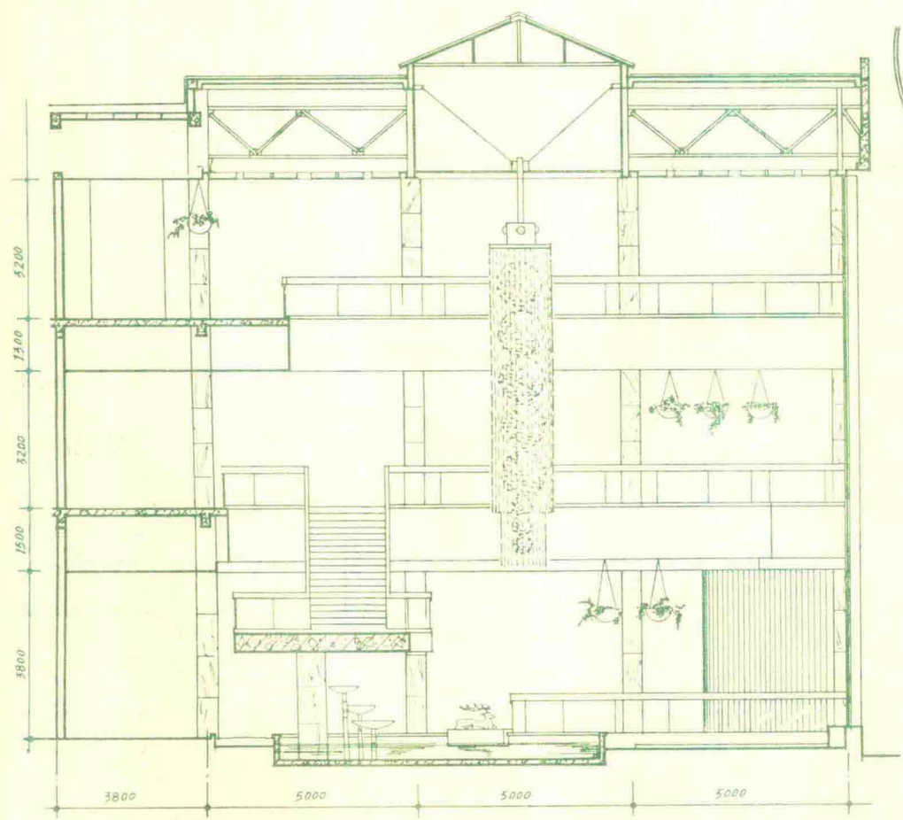
中庭剖面
