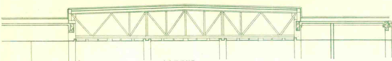
中度平頂剖面
