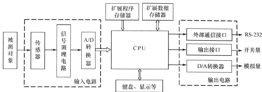
图 1.4 内嵌微处理器测试系统的结构
