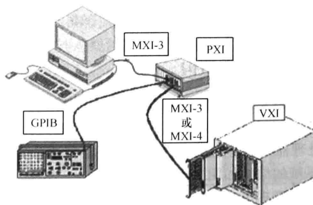
图 1.2 典型的自动测试系统组成结构
