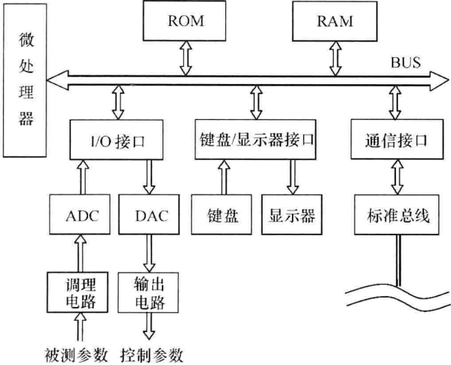
图 1.1 智能仪器的典型结构
