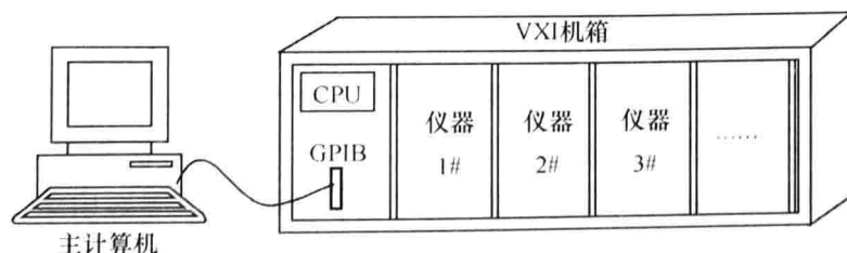
图 1.6 典型的基于 VXI 模块化仪器的个人仪器测试系统
