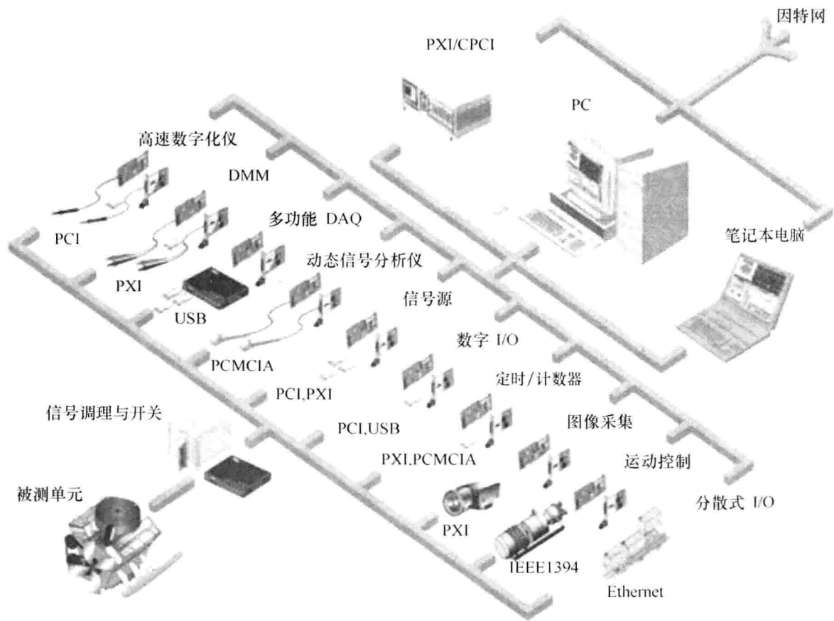
图 1.3 虚拟仪器的组成结构
