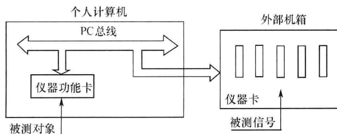
图 1.5 个人仪器测试系统结构框图
