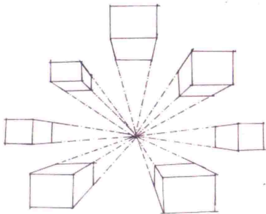
一点透视
