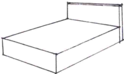
床形体演变
