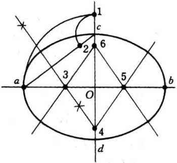
图 1-24 椭圆的近似作图法
