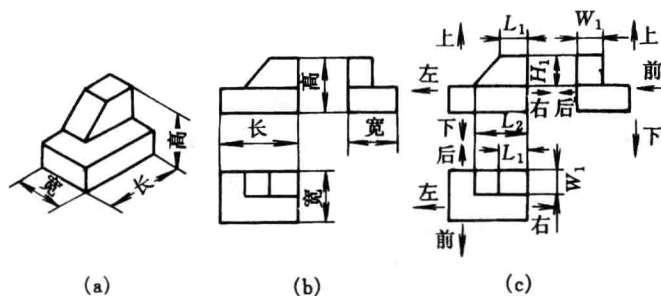
图 1-27 三视图间的长、宽、高尺寸关系
