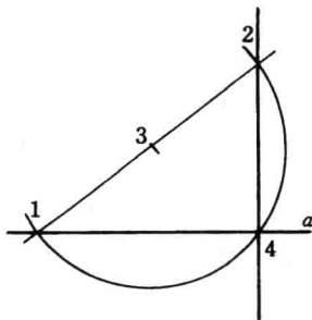
图 1-3 半圆法作垂线
