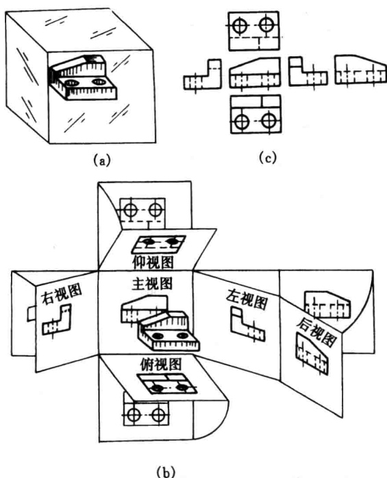
图 1-25 基本视图
