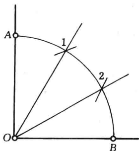
图 1-9 直角的三等分法
