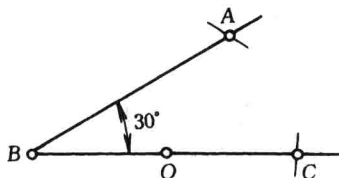
图 1-5 30^\circ 角的作法
