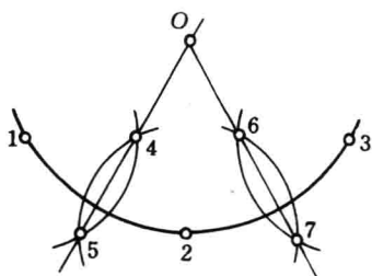
图 1-12 圆弧的作法
