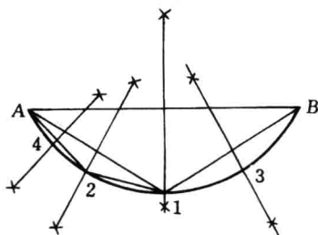
图 1-13 圆弧四等分法
