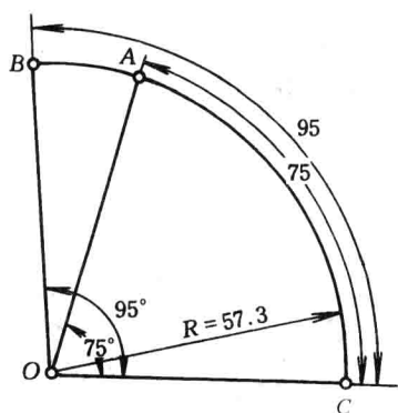
图 1-7 任意角的作法
