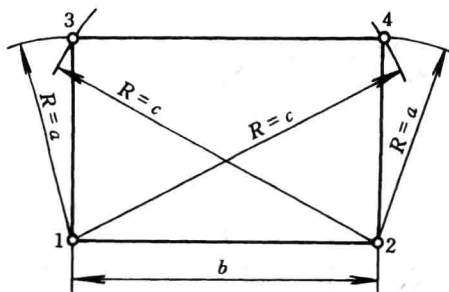
图 1-19 矩形的作法
