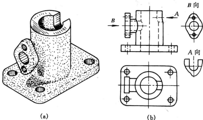
图 1-28 局部视图
