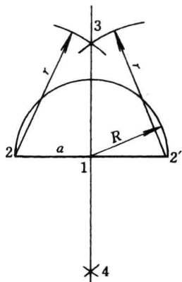
图 1-2 中垂线法作垂线
