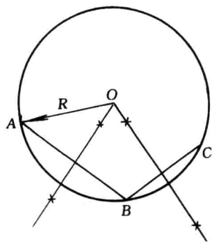
图 1-14 过三定点作圆的方法
