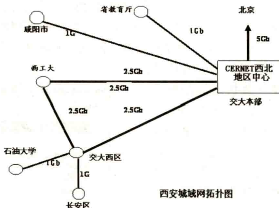
图1-11 城域网拓扑图
