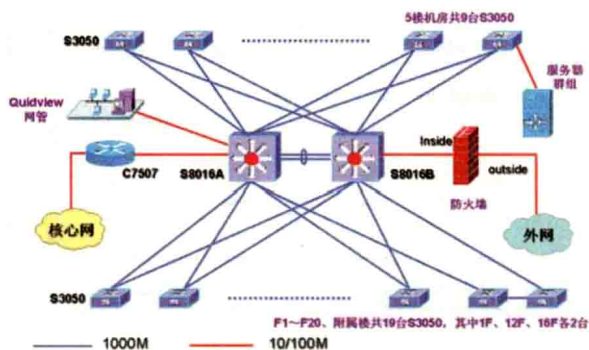
图1-10 局域网拓扑图
