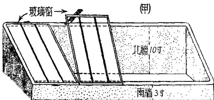
(圖五) 溫床圖稿
