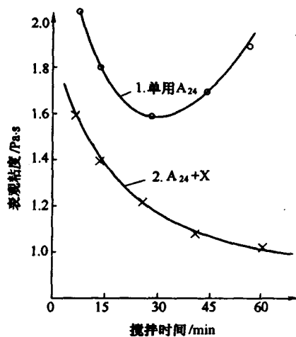
图 11-5 抗剪切试验
