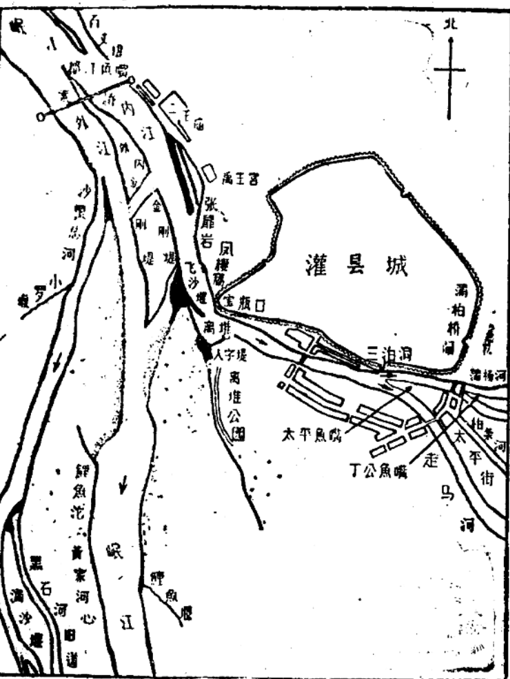
都江堰工程图
