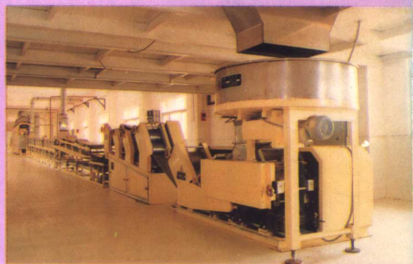
BFP-12 方便面生产线
