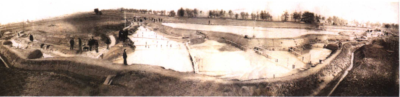
大型露天河工试验现场
