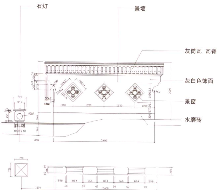
平面图(景墙石灯)
