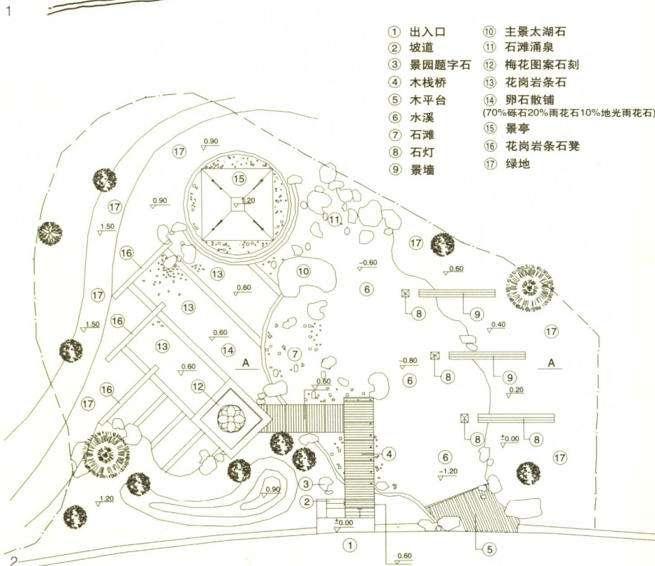
1 总平面图手绘方案
