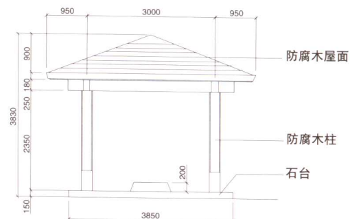
立面图
