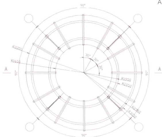
景亭平面图
