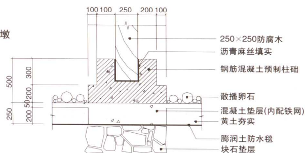
方形桥墩剖面大样图
