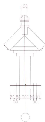
山墙脊立面图
