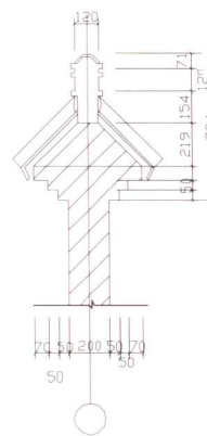
山墙脊剖面图
