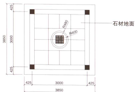
6 平面图(景亭方案二)
