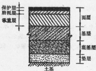
图1-2 路面结构示意图
