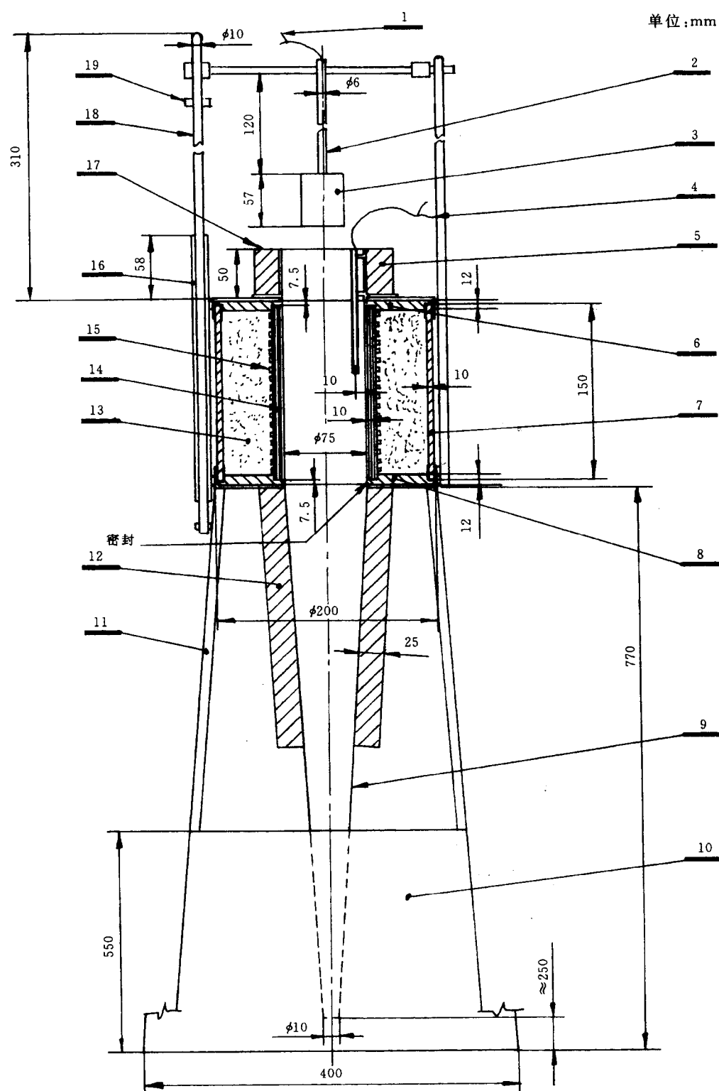
1—试样热电偶; 2—支承件钢管; 3—试样架; 4—炉内热电偶; 5—矿棉隔热层; 6—顶板; 7—石棉水泥(或类似材料)管; 8—底板; 9—空气稳流器; 10—气流屏; 11—支架; 12—矿 棉隔热层; 13—氧化镁粉; 14—耐火管; 15—加热线圈; 16—导槽; 17—气流罩; 18—插入 装置; 19—定位块
