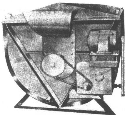
洋菇殺菁機
