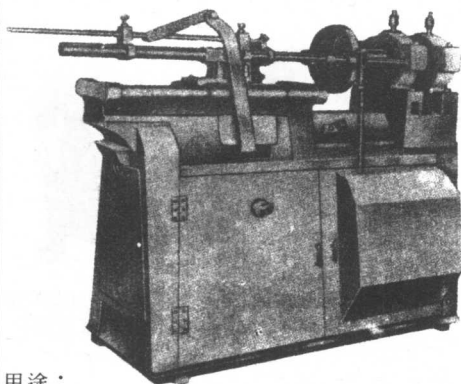
鳳梨自動剝皮去蕊機
