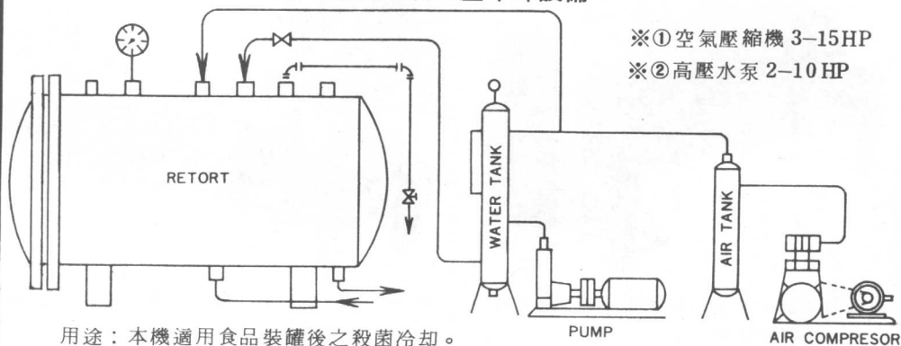
臥式殺菌釜及加壓冷却設備
