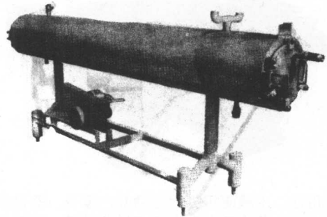
管式(熱交換器)瞬間殺菌機
