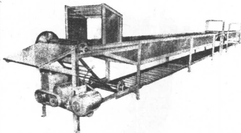
自動殺菁冷却機
