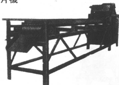
洋菇切片機
