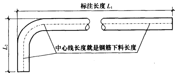
图 1-7 中心线长度
