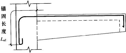
图 1-2 锚固长度
