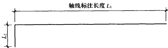
图 1-3 图纸一般标注钢筋的尺寸
