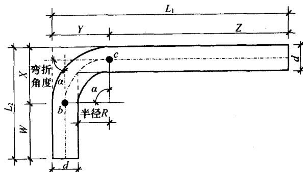
图 1-8 实际下料长度
