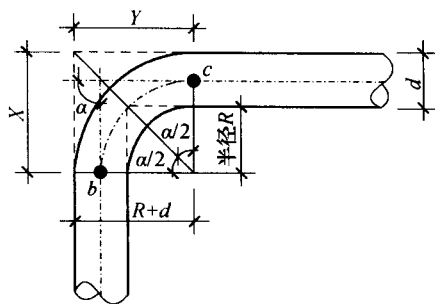
图 1-9 X、Y 的长度图
