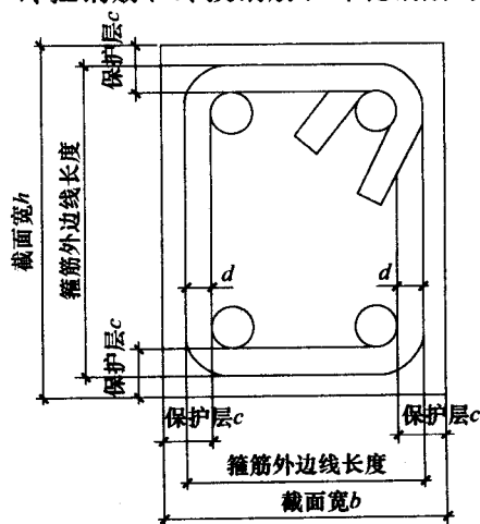
图 1-1 混凝土保护层
