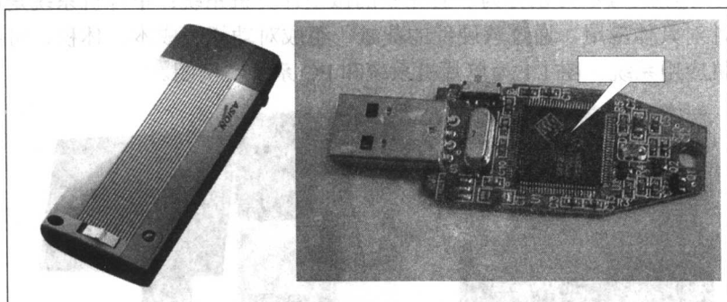
图 1.4 优盘
