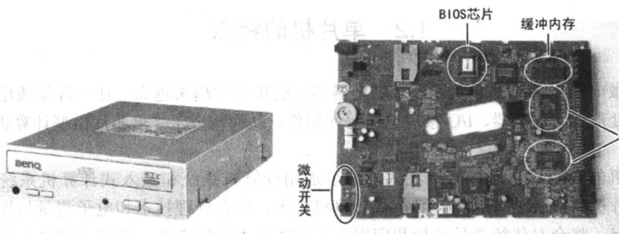
图 1.3 PC 的光驱
