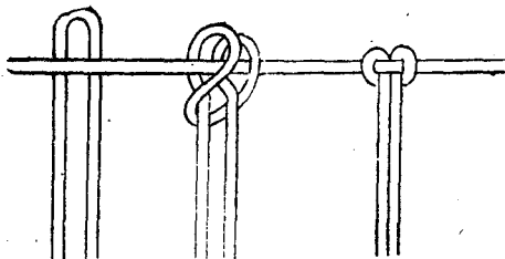
圖 16 圖 17 圖 18 內套結
