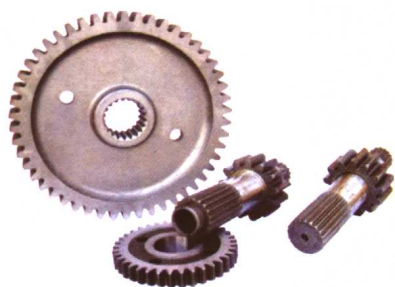
60-80 马力大型拖拉机变速箱部分齿轮
