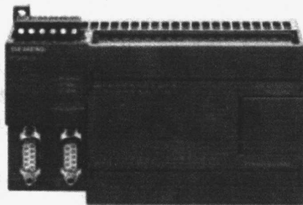
图 1-1 整体式 PLC(S7-200)的外观结构图
