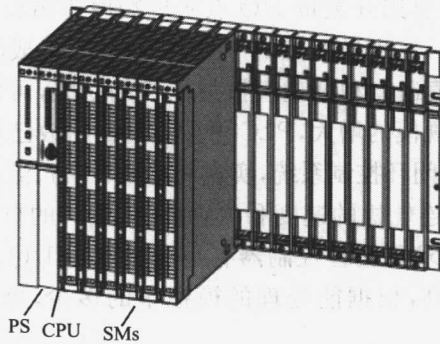
图 1-2 模板式 PLC(S7-400)外观结构图
