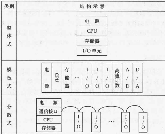
图 1-3 可编程控制器外观结构示意图
