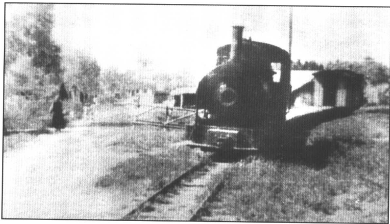
大生三厂为运输方便,在厂与长江边青龙港之间铺设火车铁路,全长 5500 米(1921 年)。
